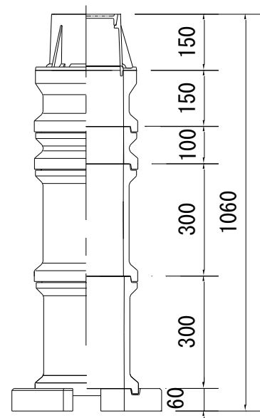
図5-7 公道部 止水栓(バルブ)ボックス仕様図
