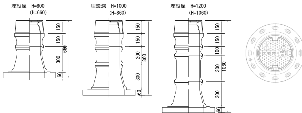
図5-3 仕切弁ボックス仕様図
